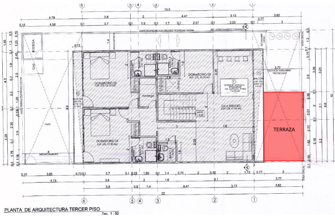
PLANTA 3° PISO
